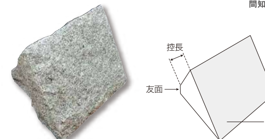
間知石
